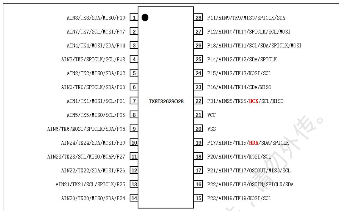
图 3 - TX8T3262S028 (SOP28) 封装图
